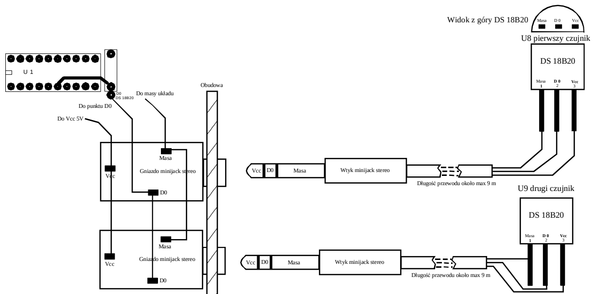
Podłączenie czujników do układu
